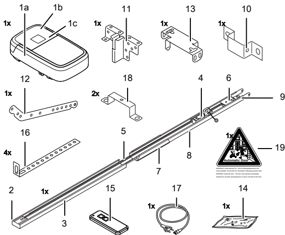
Obr. 2: Přehled produktu – jednotlivé díly
