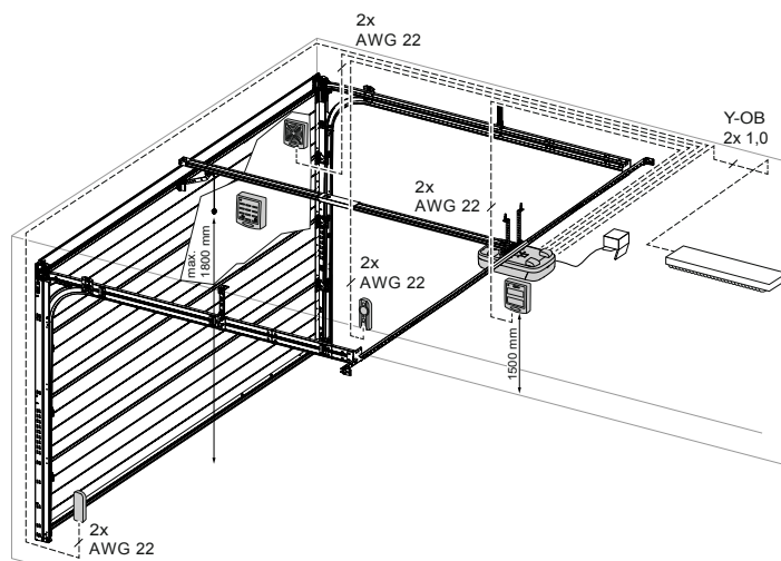
Obr. 3: Příklad instalace příslušenství
