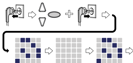
Obr. 6: Výmaz všech ručních vysílačů naprogramovaných na pohonu
