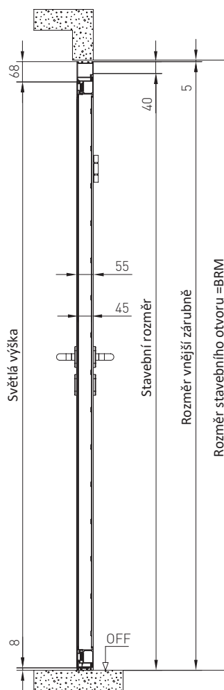
Svislý řez / Instalace do stavebního otvoru
