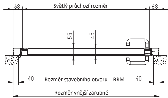
Vodorovný řez / Instalace za stavební otvor
