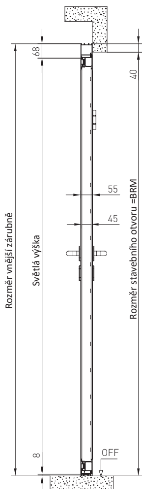
Svislý řez / Instalace za stavební otvor
