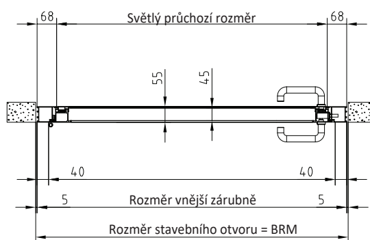
Vodorovný řez / Instalace do stavebního otvoru
